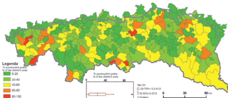
Ryc. 4. Procentowy udział zlewni podatnych na formowanie gwałtownych wezbrań w powierzchni gmin
