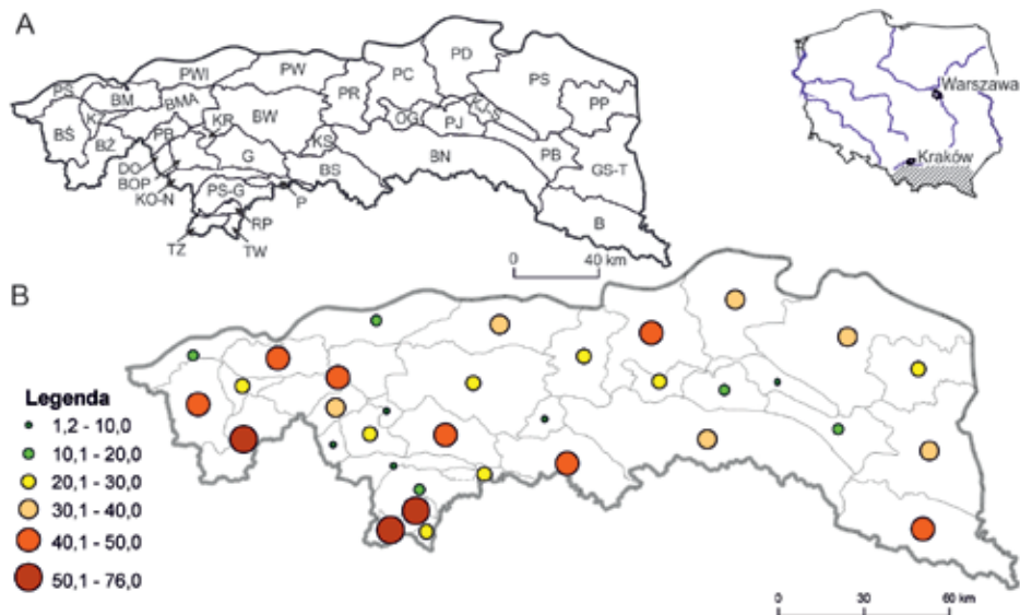
Ryc. 2. Procentowy udział zlewni w powierzchni regionu fizycznogeograficznych – A, podział Karpat na regiony fizycznogeograficzne – B (Bryndał 2014b)
