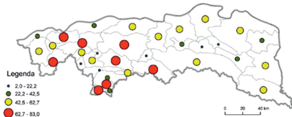
Ryc. 3. Przestrzenne zróżnicowanie wskaźnika podatności terenowej Wpt w regionach fizycznogeograficznych (Bryndał 2014b)
